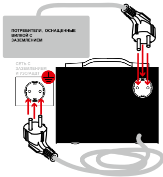
Схема подключения стабилизатора в сеть с заземляющим проводом и УЗО
