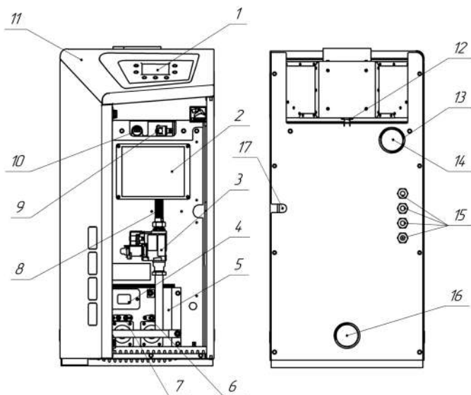
Рис. 1. Конструкция котла.
