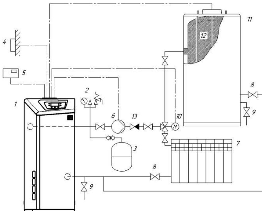
Рис. 5. Примерная гидравлическая схема подключения котла к системе отопления и бойлеру косвенного нагрева с разделительным клапаном*
