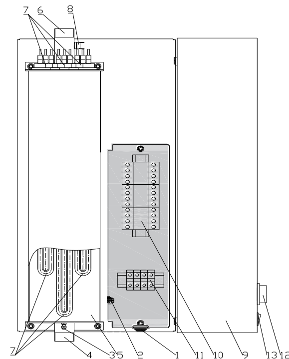
Рисунок 1. Устройство электрокотла. (крышка открыта)
