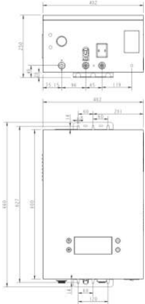
Рис.2. Габаритные размеры
