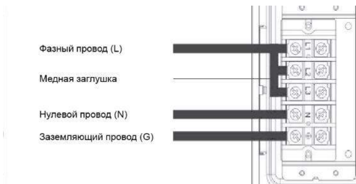
Рис. 8. Однофазное подключение прибора – зеркальный порядок
