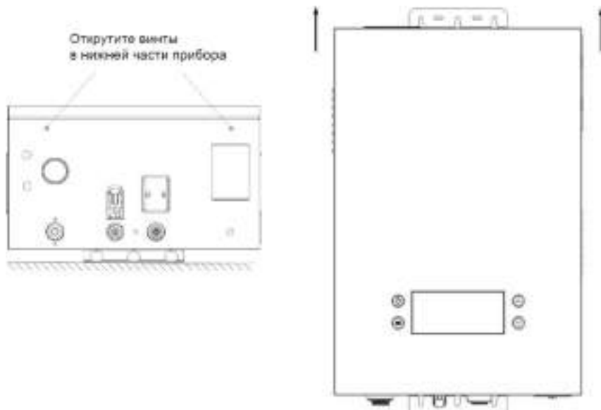
Рис. 7. Демонтаж лицевой панели
