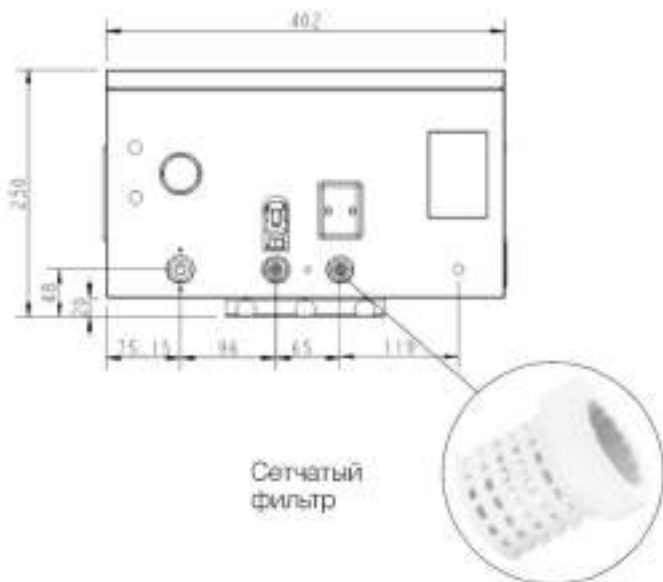
Рис. 13. Сетчатый фильтр
