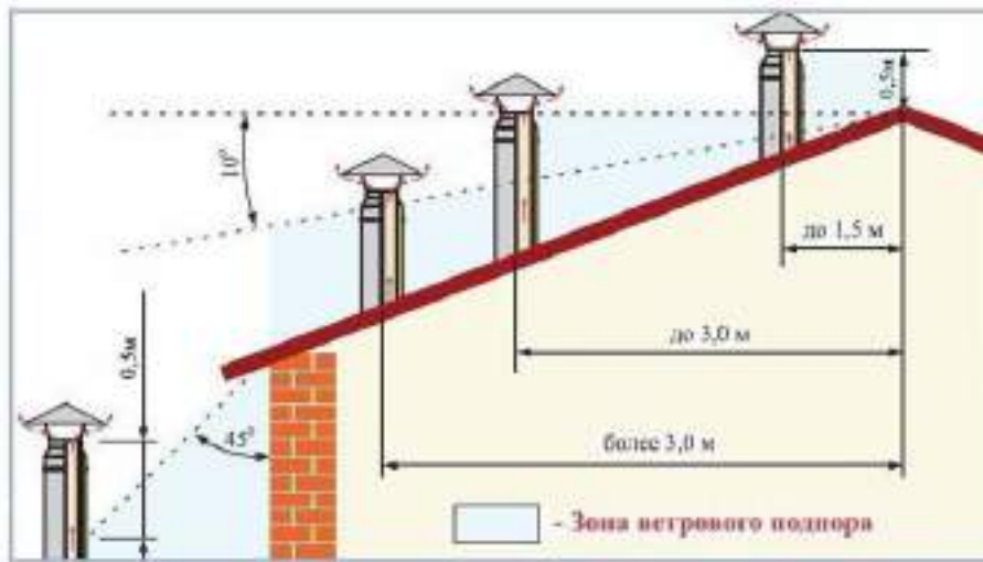
Рис. 7 Высота дымохода.
